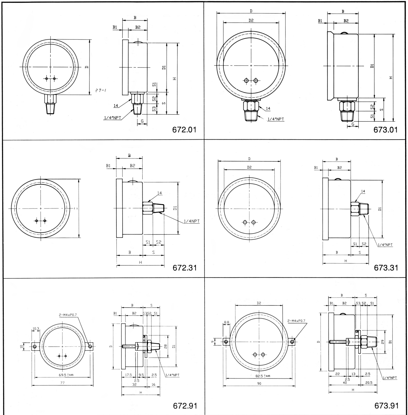
外觀尺寸規格 (mm)
